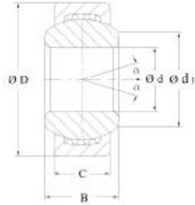
GEG..E GEG..ES
